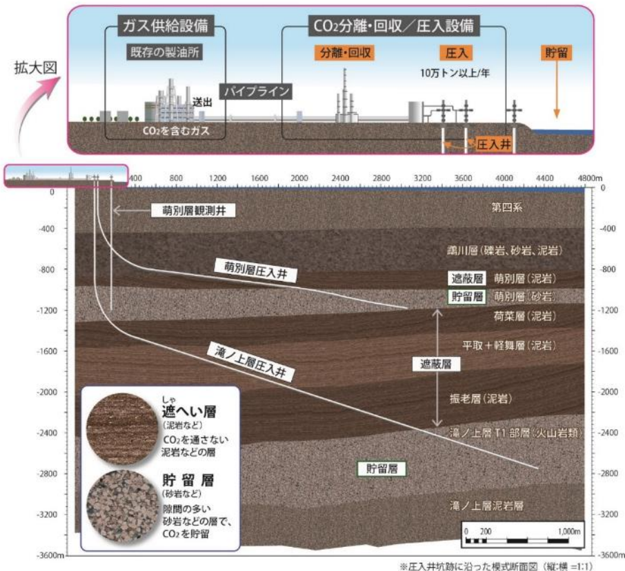
苫小牧CCS実証試験の全体像
