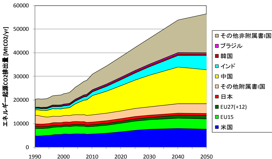
図 1 世界主要国・地域別のエネルギー起源 CO 2 排出見通し (2008 年までは IEA 統計値 8) )
