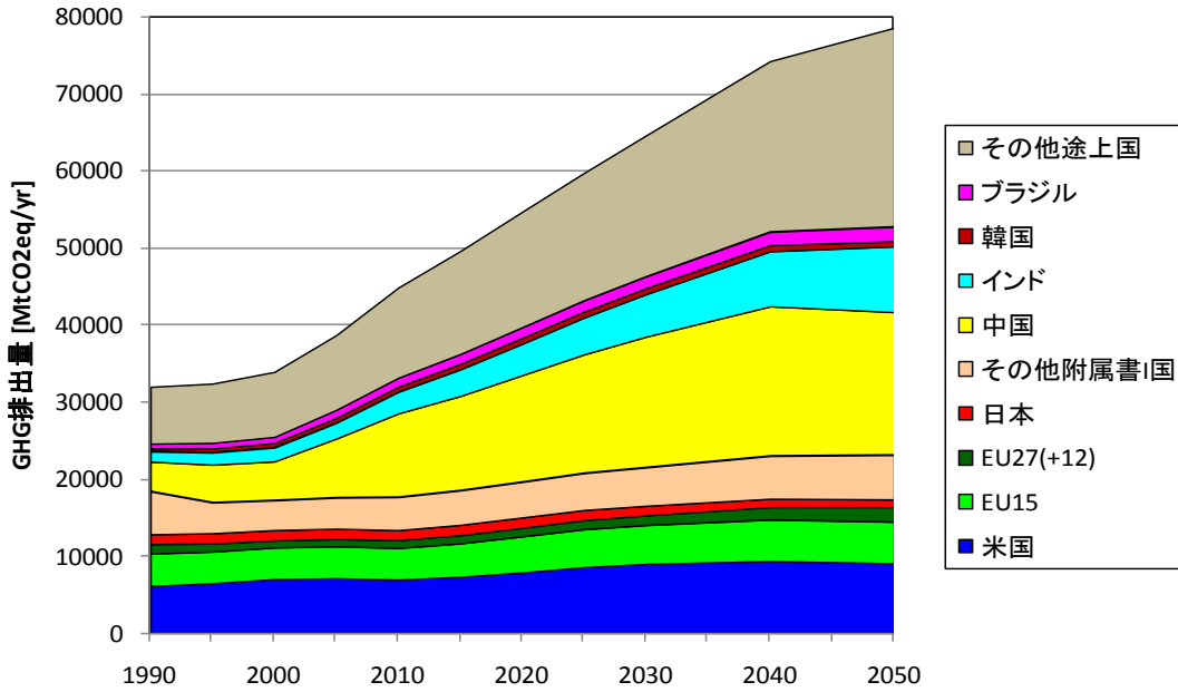
図3 世界主要国・地域別の GHG 排出見通し (2005 年までは附属書 I 国 : UNFCCC 9) 、非附属書 I 国 : IEA 統計値 8) )
