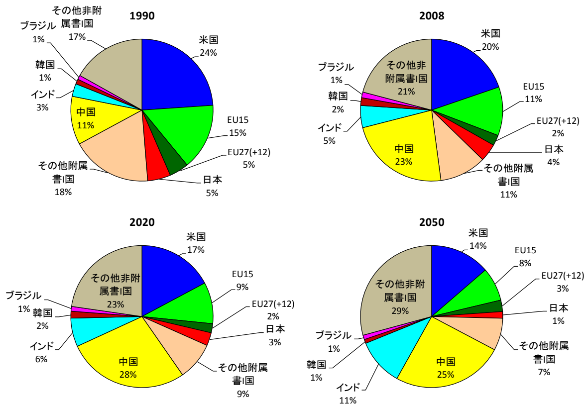
図2 エネルギー起源 CO 2 排出の各国シェア (1990、2008 年は IEA 統計値 8) 、2020、2050 年は RITE 推計値)
