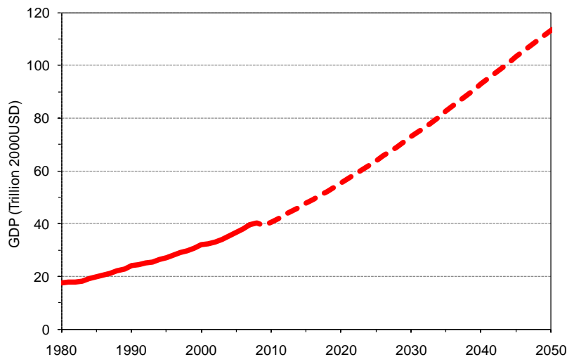
付図 4 世界の GDP 見通し （実線：統計、破線：推計）
