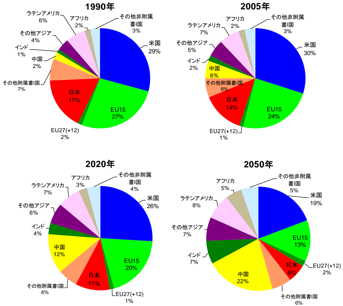
付図5 GDPの各国シェア
