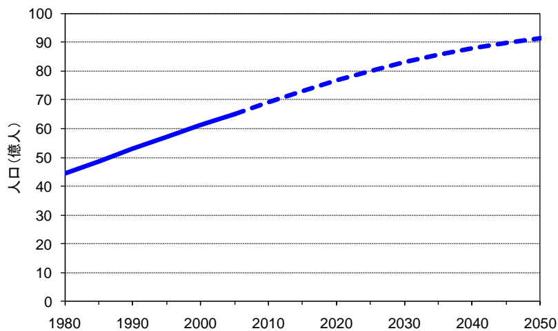
付図 3 世界人口の見通し（国連 2008 年中位推計） （実線：統計、破線：推計）
