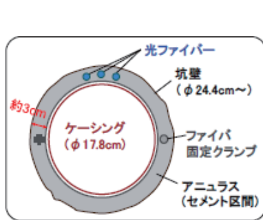
光ファイバーの設置概念図
